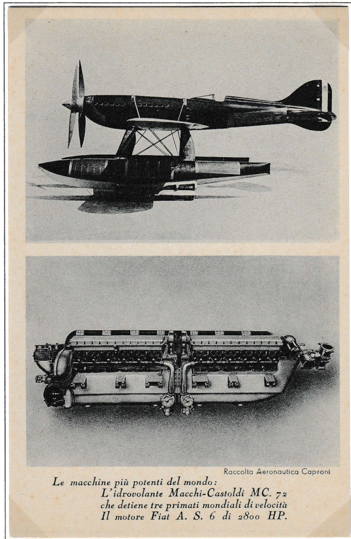
Idrovolante Macchi-Castoldi M.C.72 e motore Fiat A.S.6 da 2800 HP
