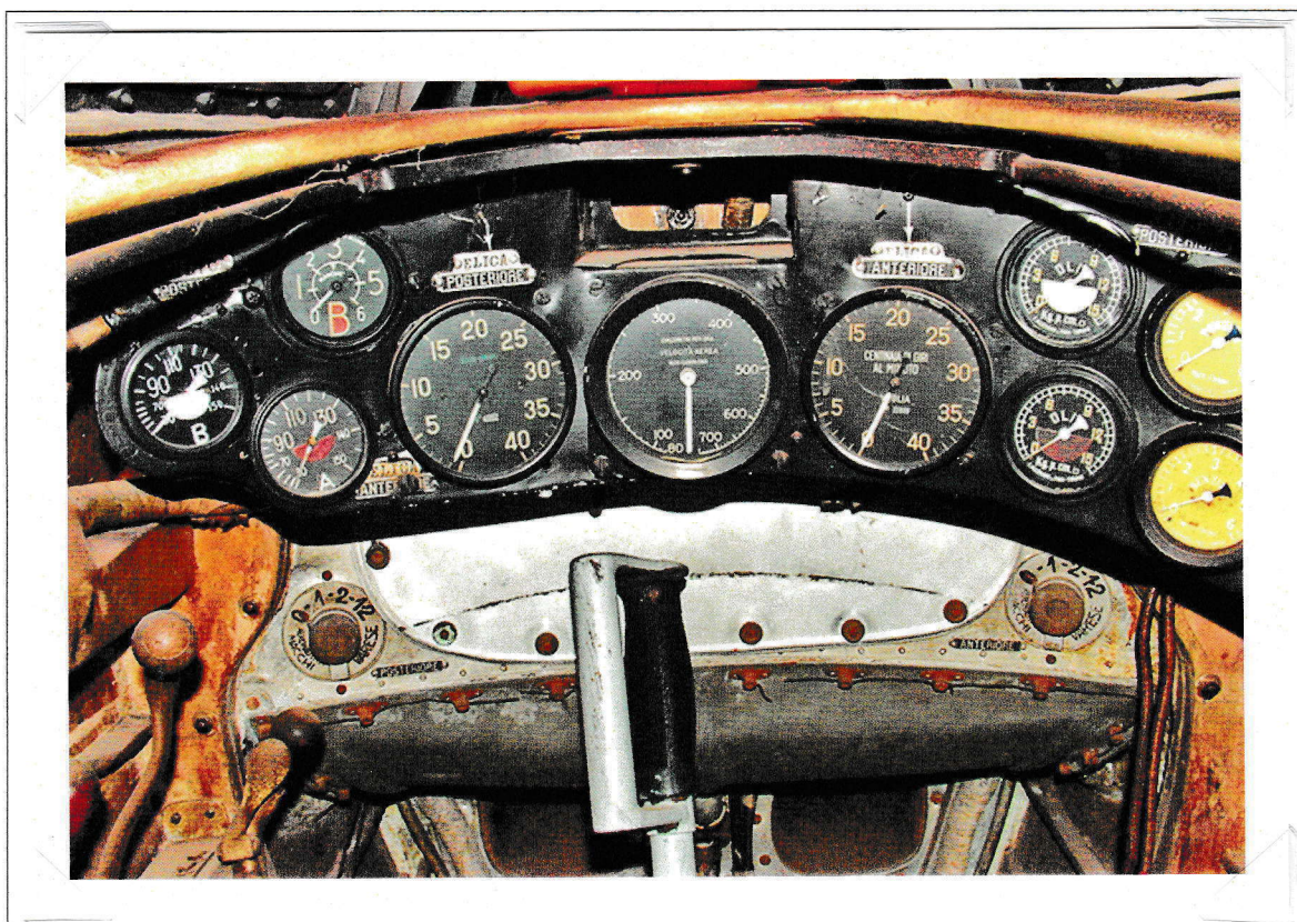
Particolare dell'abitacolo del M.C.72
